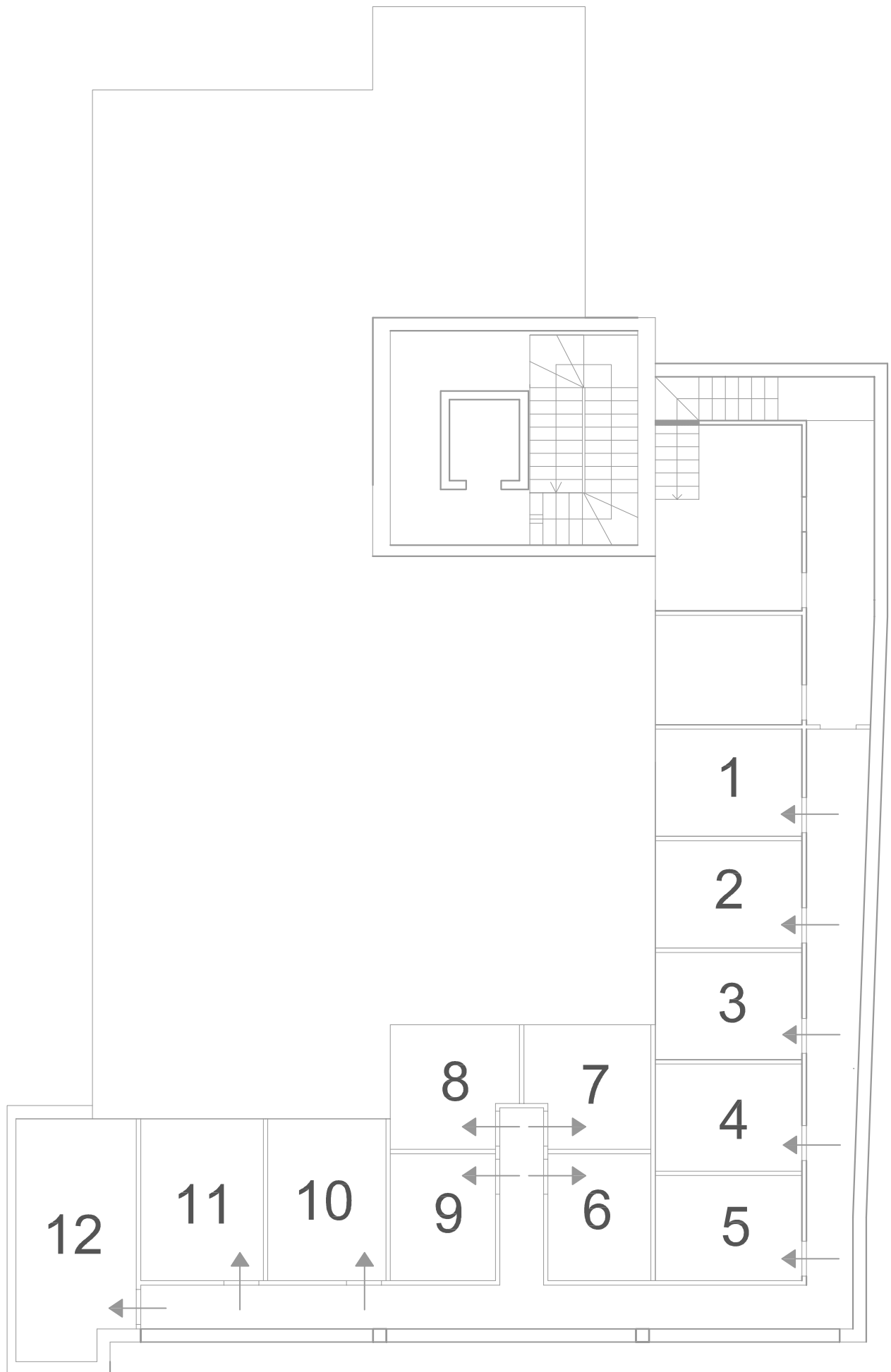
PIANO 1° INTERRATO
